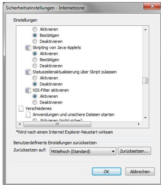
Abb. 9: Dialog Sicherheitseinstellungen
