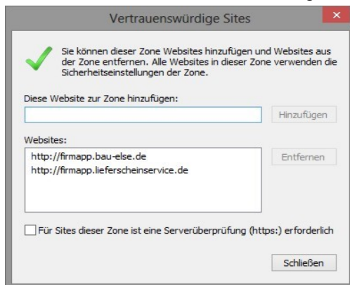
Abb. 8: Seite hinzugefügt
