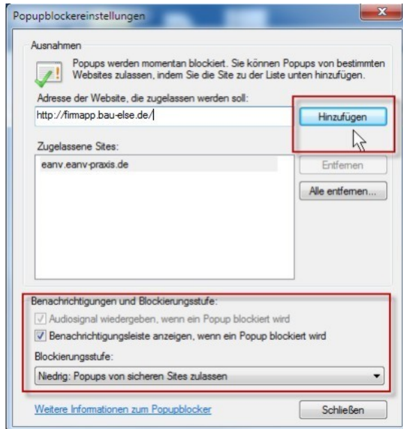
Abb. 10: Dialog Popupblockereinstellungen
